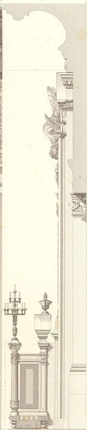
Coupe sur la ligne A.B. Fig. 3.
