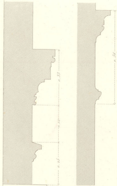
Profil D. Fig. 5.
