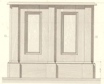
Coupe sur la ligne GH
