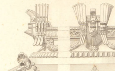
Pavillon d'entrée des Abonnés Détails de l'amortissement du Dôme
