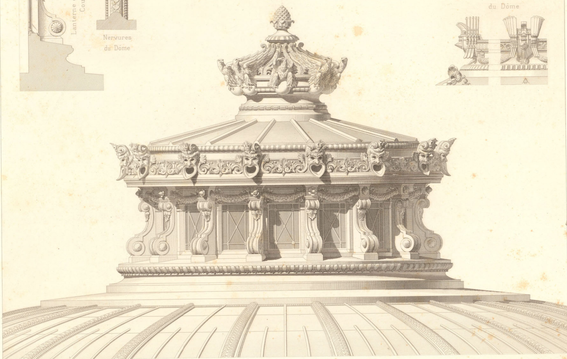
Pavillon d'entrée des Abonnés Détails de l'amortissement du Dôme
