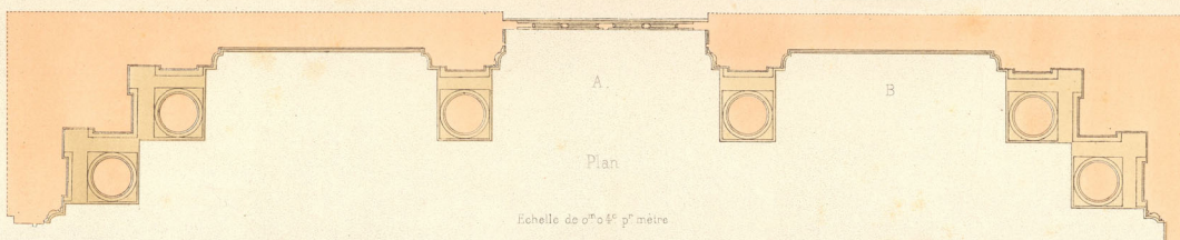
Détail de la fenêtre A et du mur B
