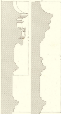
Profil du Meuble Colonnettes F. Pilastres G. Fig. 7. Fig. 8.
