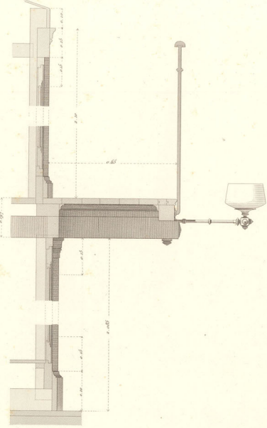
Détails des Armoires Coupe sur IJ.
