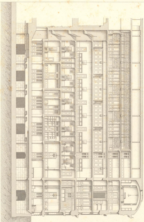
Coupe passant par la Salle des Choristes (Femmes) (Voir le plan Pl. 10.11)
