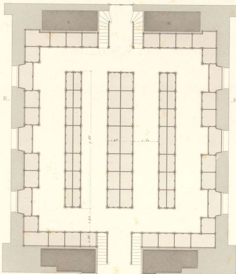
Plan à la hauteur de AB.
