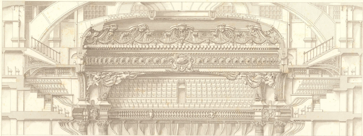
Coupe suivant AB (Côté de la Salle)
