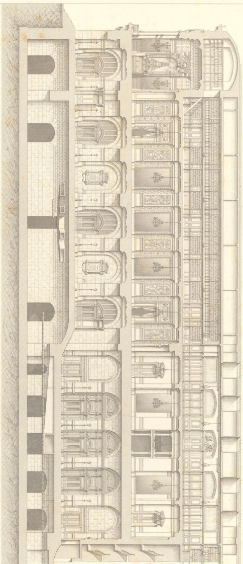
Coupe passant sur la Galerie du Glacier (Voir le plan Pl. 10.11)
