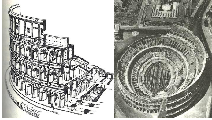
Şekil 4.23 Flavian Amfitiyatrosu (Colloseum), Roma, İtalya. M.S. 80 (Roth, 2006)
