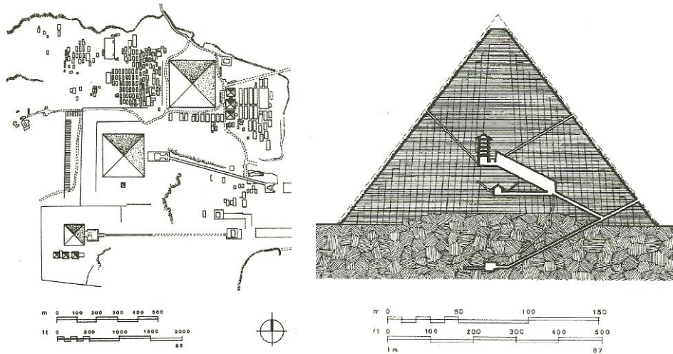
Şekil 4.11 Giza Piramit Grubunun planı ve Khufu Piramitinin kesiti. Kesit, tasarımdaki değişiklikleri gösterir. Mezar odası iki aşamada, en alttan kütlelin ortasına kadar taşınmıştır. (Roth, 2006)
