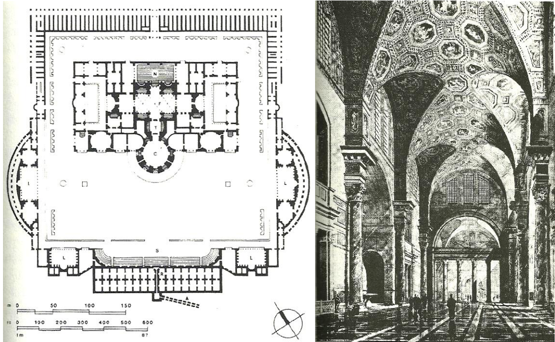
Şekil 4.24 Caracalla Hamamı, Roma, M.S. 212-216. Hamam ve çevresini gösteren plan ve iç perspektif. (Roth, 2006)
