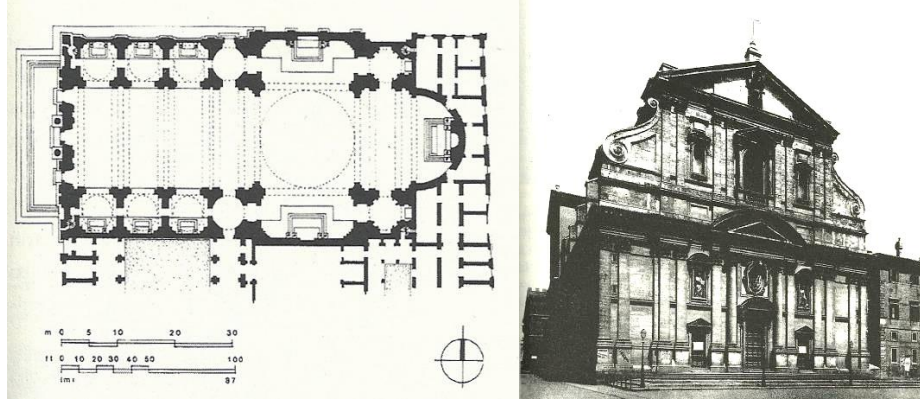
Şekil 4.37 Gesu Kilisesi, Roma, İtalya, 1568-1577. Plan ve görünüş. (Roth, 2006)
