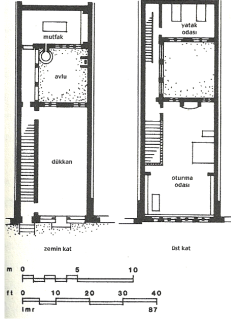
Şekil 4.31 Tüccar evi, Cluny, Fransa, 12. yüzyıl. Plan. (Viollet-le-Duc tarafından yeniden yapılmıştır) (Roth, 2006)
