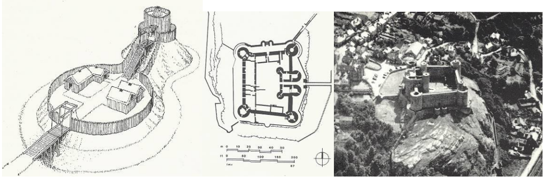
Şekil 4.27 En solda; bir motte ve bailey kalesi, 8. Yüzyıl, ortada; Harlech kalesi, Merionetshire, Galler, 1283-1290, plan, en sağda; Harlech kalesi, görünüş. (Roth, 2006)
