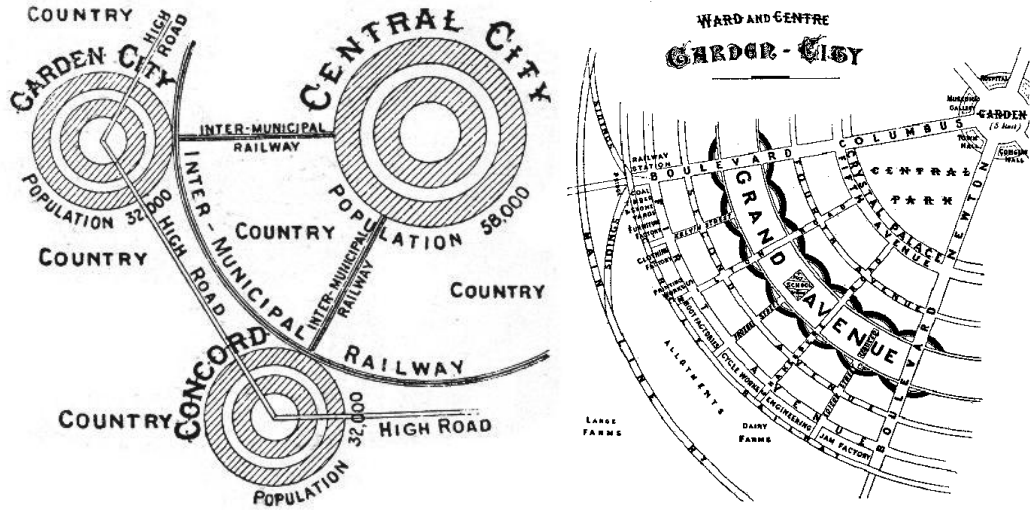
Şekil 4.53 E. Howard, Garden City çizimleri. ( http://yourdevelopment.org ), ( www.palmhaven.info )
