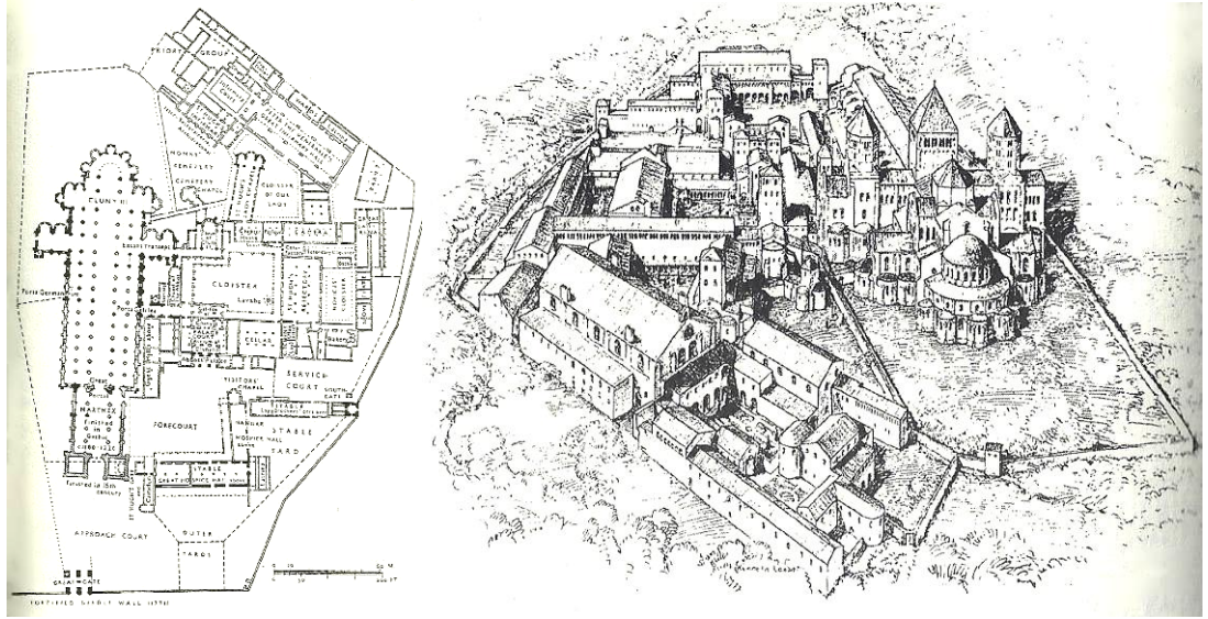
Şekil 4.28 Gunzo, III. Cluny Manastırı, Cluny, Fransa, 1088-1130. Plan ve Kenneth Conant'a ait kuşbakışı perspektif. (Roth, 2006)
