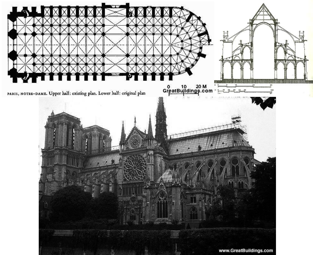
Şekil 4.29 Notre Dame de Paris Kilisesi, Paris, Fransa, 1163-1250. Üstte Solda; Plan. ( www.greatbuildings.com ) Üstte Sağda; Kesit (Roth, 2006) Alttaki; Görünüş. ( www.greatbuildings.com )
