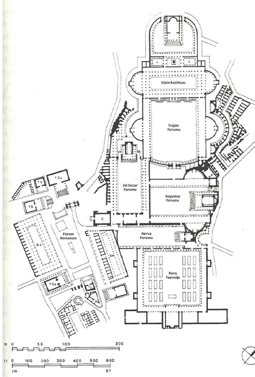
Şekil 4.19 Forum Romanum ve İmparator Forumları, Roma, M.Ö. 54-M.S. 117 arası. Birleşik İmparator Forumları, Roma kent ve politik yaşamının merkezi eski Forum Romanum bitişiğinde, girift eksenler üzerinde birbirini izleyen imparatorlar tarafından yaptırılmıştır.
