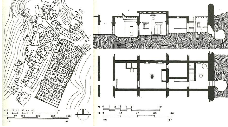
Şekil 4.12 Deir el-Medineh, Mısır, M.Ö. 1530 civarı. Genel yerleşim planı ve bir zanaatçı evine ait plan ve kesit. Ön cephedeki kabul odası, ana oda, yatak odası ve açık mutfakıyla Mısır evinin temel bileşenlerini göstermektedir. (Roth, 2006)
