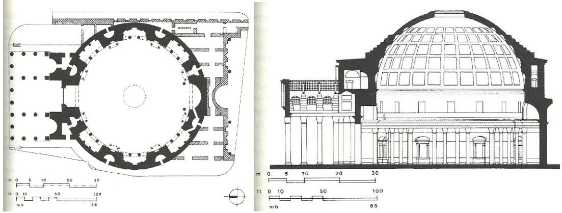
Şekil 4.20 Pantheon, Roma, M.S. 118-128. Plan ve kesit. (Roth, 2006)
