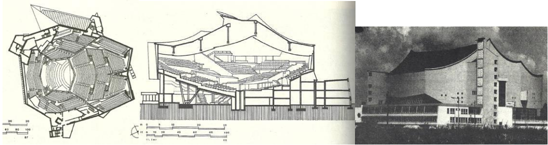
Şekil 4.51 Hans Scharoun, Berlin Filarmoni, 1957-1965. Binanın olağandışı planı ve profili, müziği dinleyicilerin ortasına yerleştirme isteğiyle şekillenmiştir. (Roth, 2006)
